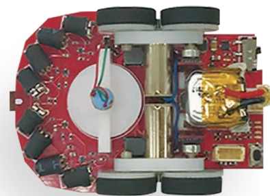
<原寸> 2017～2019年マイクロマウス競技優勝機 「Fantom2nd (松井 祐樹氏)」 長さ 52mm×幅 38mm×高さ 20mm 重量 11.8g
